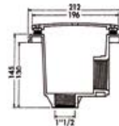
Zijopening 1" 1/2 of 2" te schroeven bodemopening met schroefdraad 1"1/2 met doorslagdeksel
