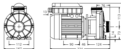
Centrale aanzuigpomp
