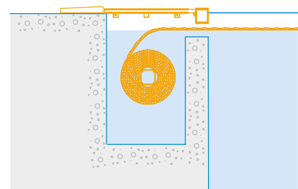
Gemetselde tussenwand
