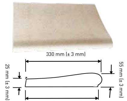
Randsteen recht
