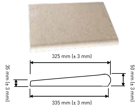
Randsteen recht
