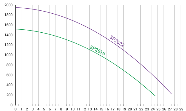
Koppelingen 63 mm
